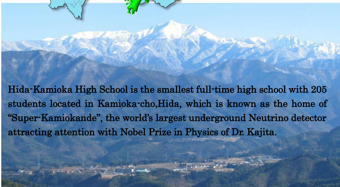
Super-kamiokande
