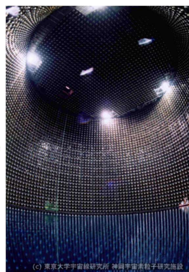
Super-kamiokande
