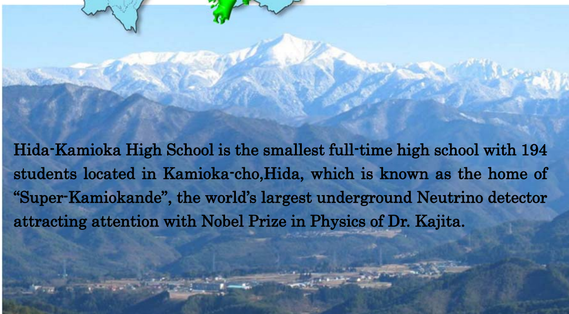
Super-kamiokande
