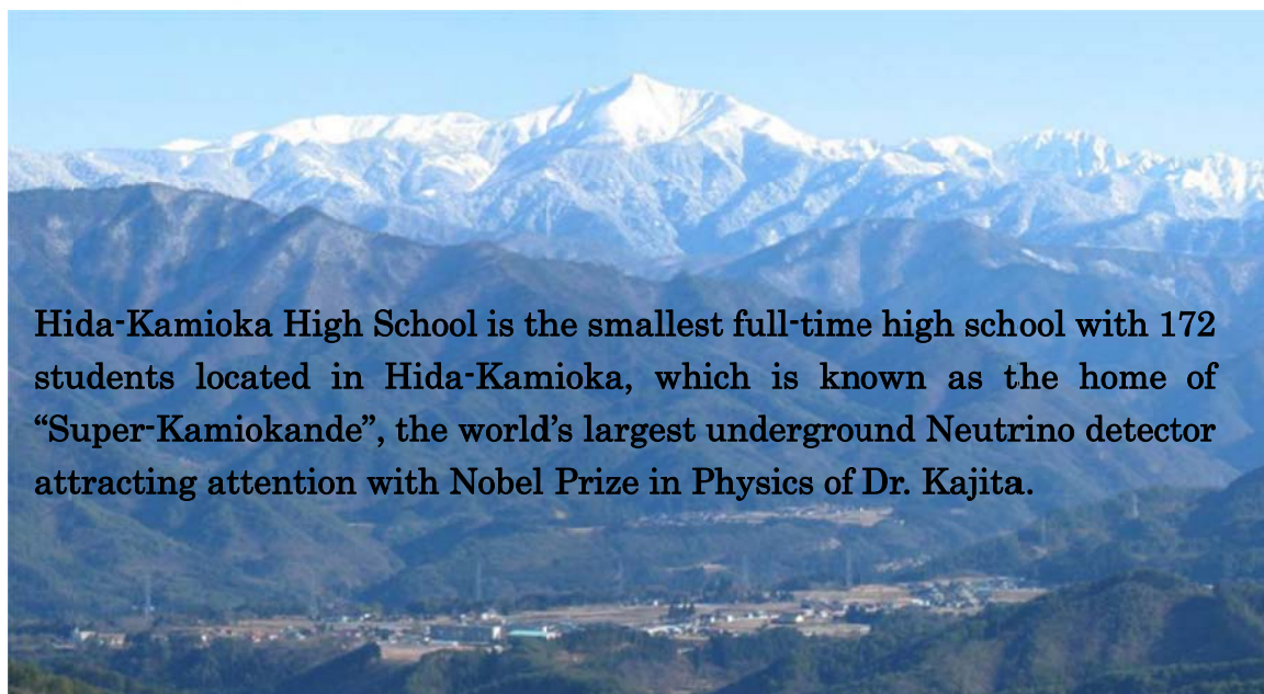
Super-kamiokande
