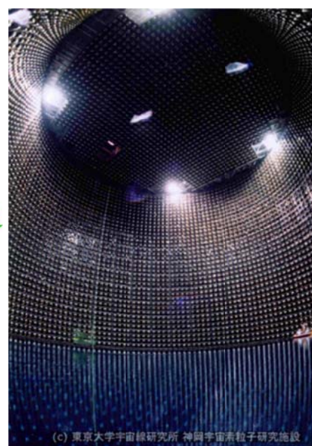
Super-kamiokande
