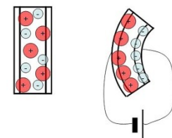
高分子アクチュエータの駆動機構のモデル
